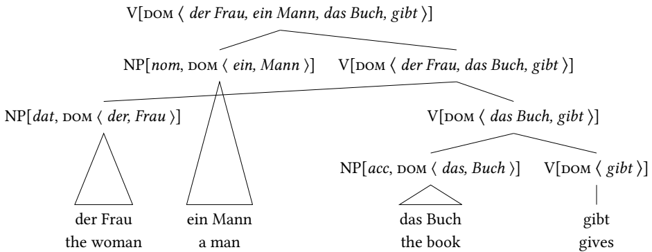
Figure 11.39: Analysis of dass der Frau ein Mann das Buch gibt ‘that a man gives the woman the book’ with binary branching structures and discontinuity
